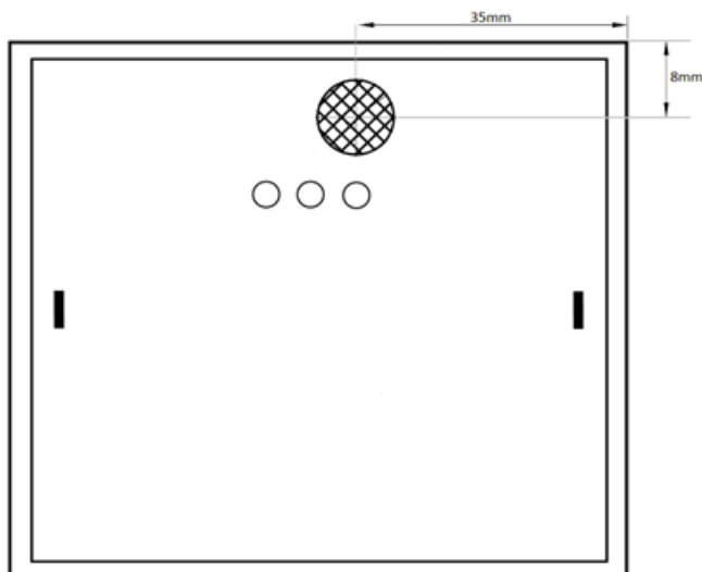
Obr. 6: Umístění magnetu
