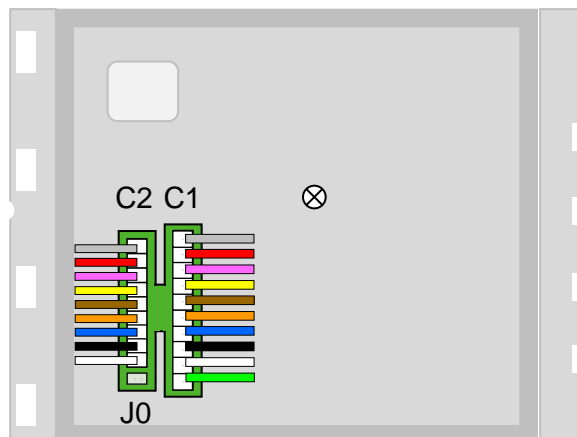
Obr. 2: Zadní strana čtecího modulu MREM 58 SferON
